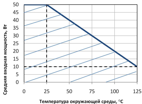
Нагрузочная кривая
