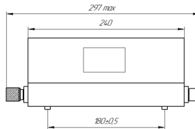
ПР1-25-500-2 (масса, не более: 3,8 кг)
