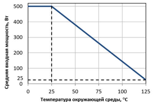
ПР1-25-500-2 (масса, не более: 3,8 кг)
