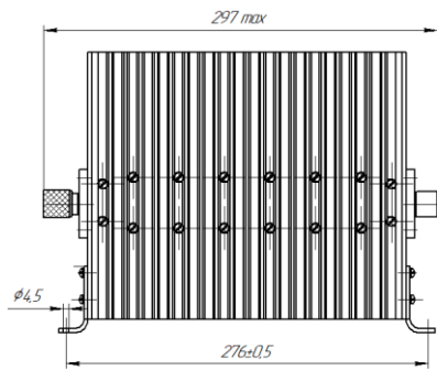
ПР1-25-500-1 (масса, не более: 5,9 кг)
