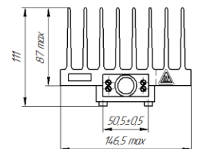
ПР1-25-500-2 (масса, не более: 3,8 кг)
