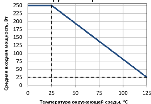
Нагрузочная кривая
